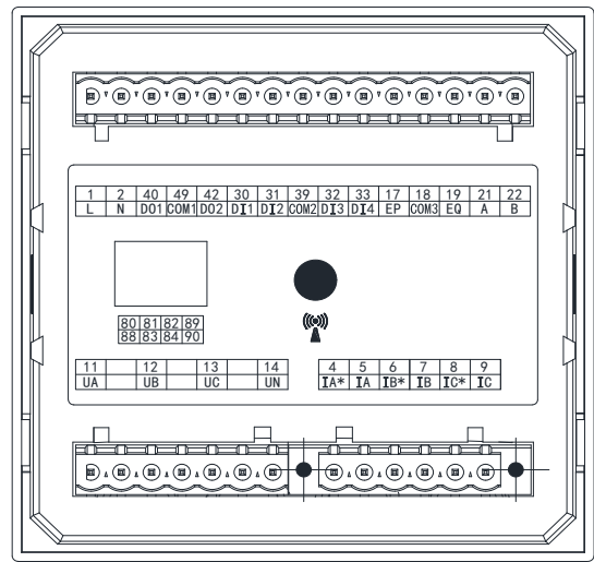
图 18 DEMPSeries AC3-D92 扩展 WF/LoRa 接线图
