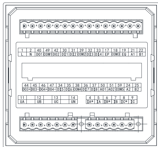
图 14 DEMP-AC3-D92 扩展 K/2M/2C
