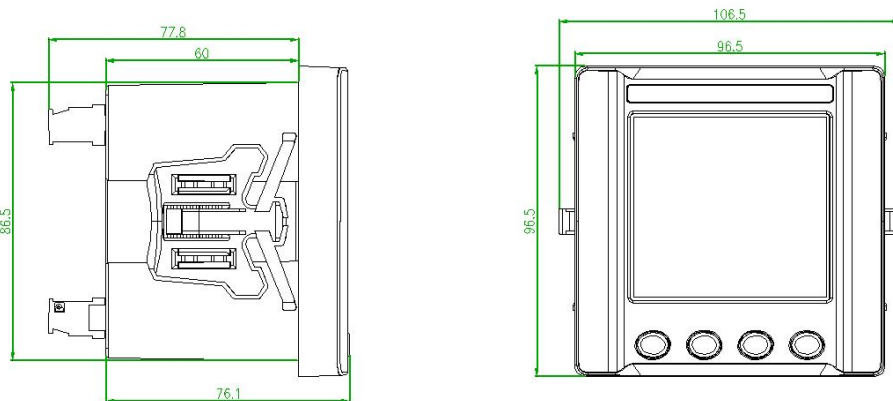
图 3 DEMP-AC3-D92 尺寸图
