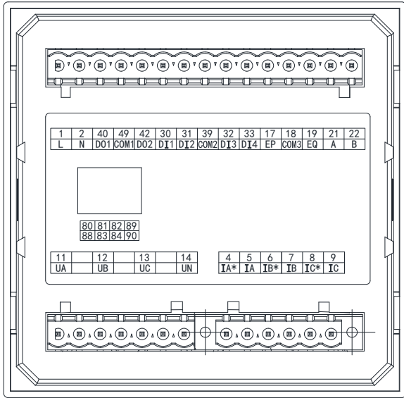
图 15 DEMPSeries AC3-D92 扩展测温/漏电接线图
