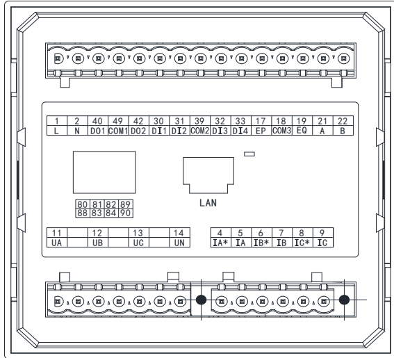
图 17 DEMPSeries AC3-D92 扩展 CE 接线图
