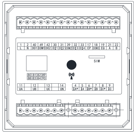
图 16 DEMPSeries AC3-D92 扩展 4G 接线图
