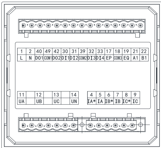
图 13 DEMP-AC3-D92 基础款接线图
