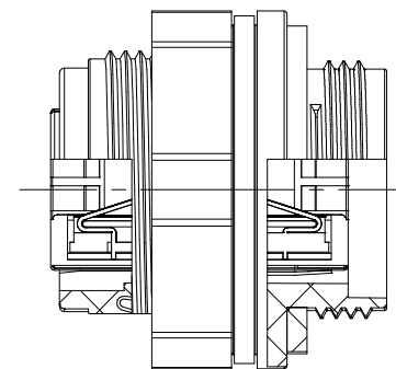
02 局部剖视图
